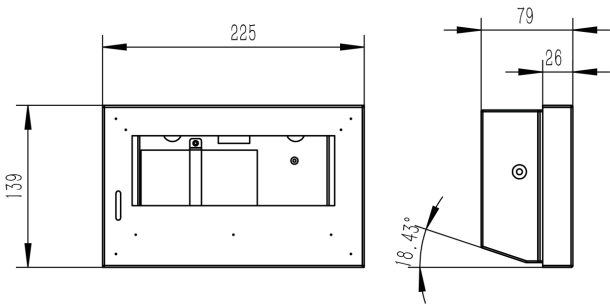
T22 / T22-S 称重显示器
